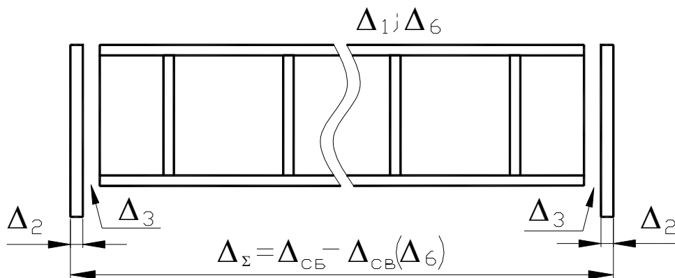
Рисунок А.1 – Схема балки
