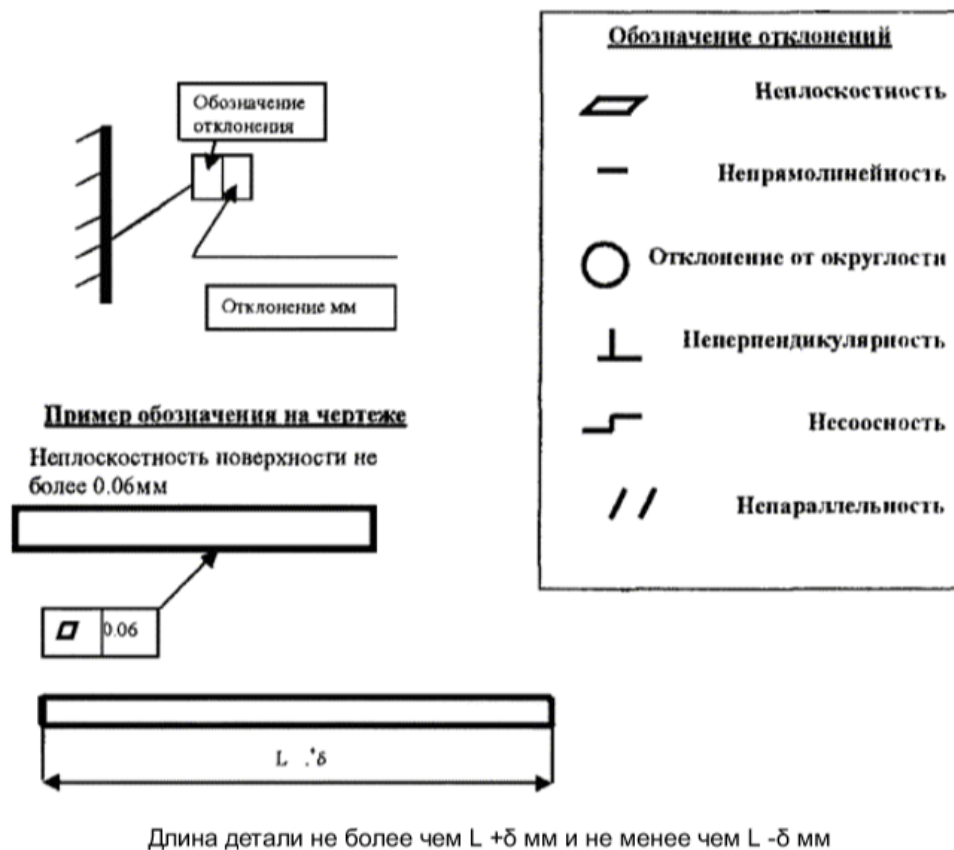
Рисунок 2 - Обозначение на чертежах предельных отклонений размеров и формы элемента
