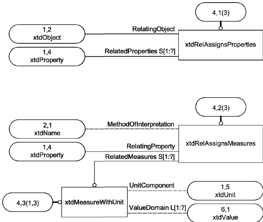
Рисунок 4 - EXPRESS-G диаграмма 4 - Назначение свойств и единиц измерений
