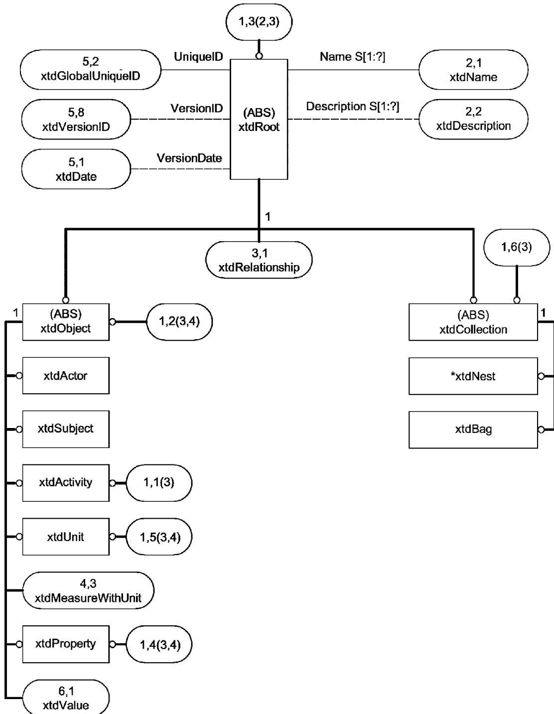
Рисунок 1 - EXPRESS-G диаграмма 1 - Верхний уровень с корневой концепцией
