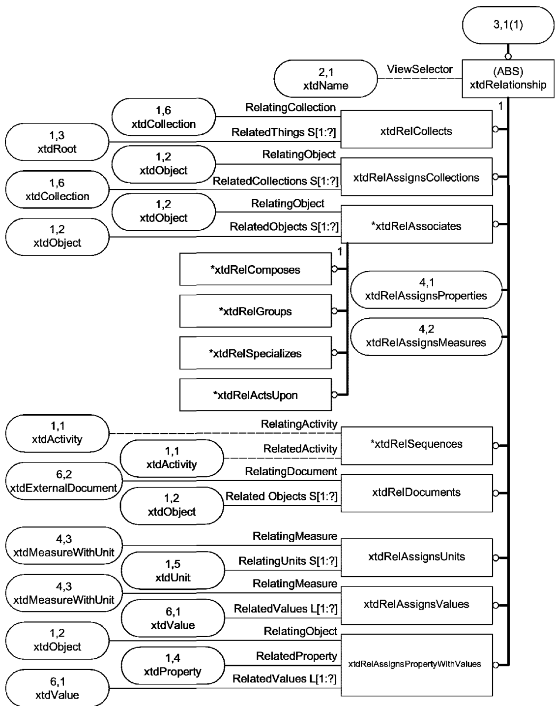
Рисунок 3 - EXPRESS-G диаграмма 3 - Отношения
