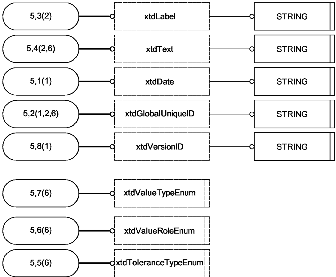
Рисунок 5 - EXPRESS-G диаграмма 5 - Основные типы
